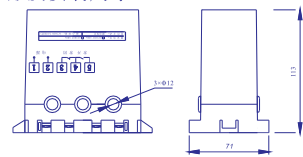
JD-5、JD-5B外形尺寸图
