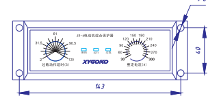
JD-6安装尺寸图
