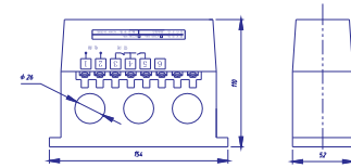
JD-6外形尺寸图
