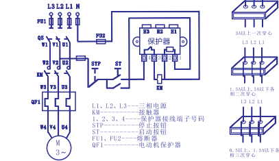
保护器工作电压为AC220V；控制电路电压为AC220V。
