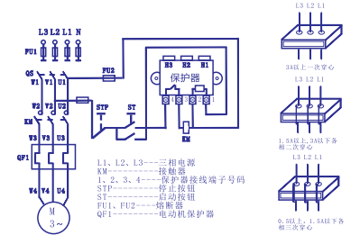
保护器工作电压为AC380V；控制电路电压为AC380V。
