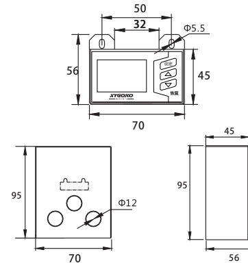
JS-50C 外形及安装尺寸图
