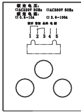
JS-50C 控制器接线图
